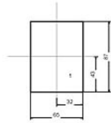
1 Türanschnitt Kiphebel ohne Blendrahmen 2 Türanschnitt Kiphebel mit Blendrahmen
